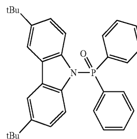
tBuCzPO
