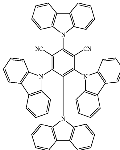
4CzIPN
